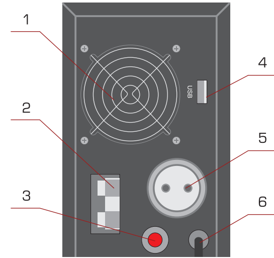
Рис. 3 Задняя панель ДБЖ
